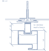
Schnitt F-F
